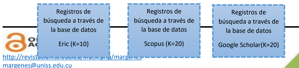
Figura 1. Diagrama PRISMA
