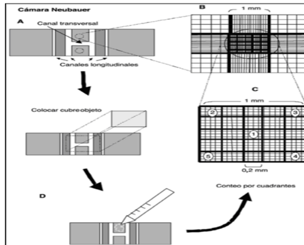
Figura 2. Procedimiento del recuento de esporas.
