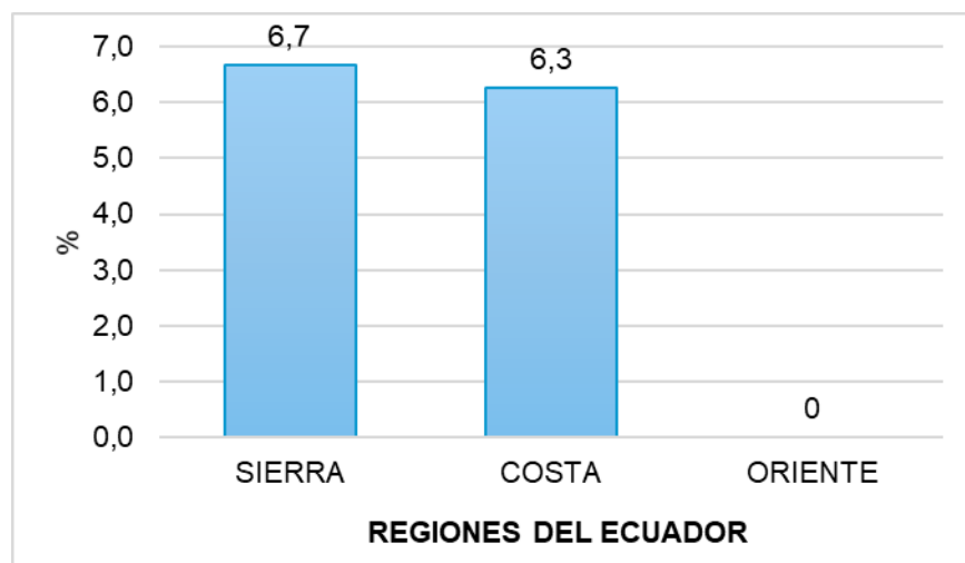
Figura 5. Prevalencia de Vairimorpha en tres regiones del Ecuador (ecotipos).
